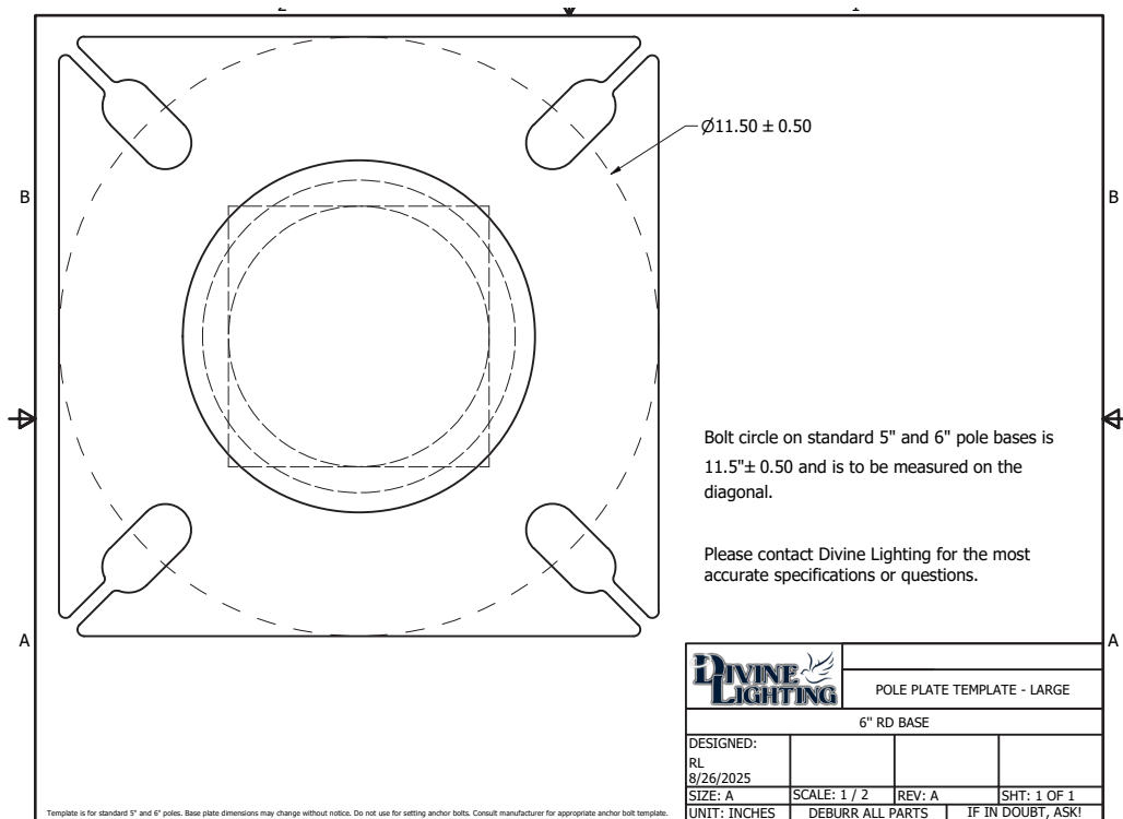
5" & 6" Pole Template
