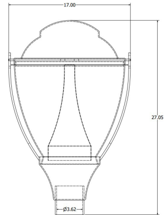
Pattern 1 & 2 Dimensions
